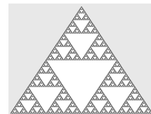
フラクタル図形の一種 (シェルピンスキーのギャスケット)
